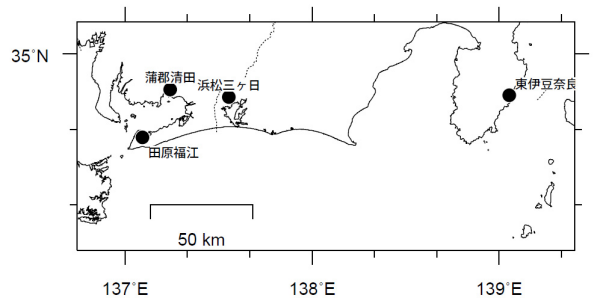
体積ひずみ計の配置図
