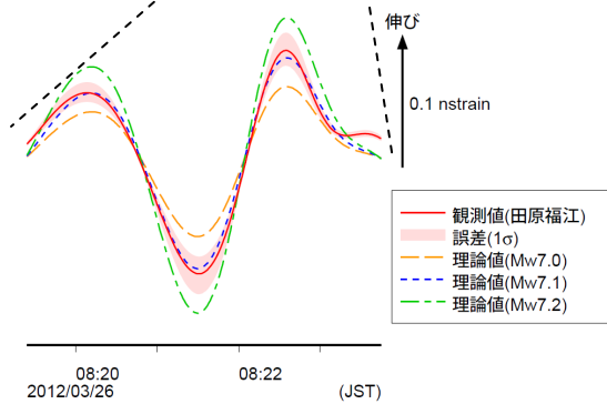
田原福江観測点の観測波形と理論波形の振幅比較 (上図) データには周期 120~333 秒のバンドパスフィルタを時間軸の正逆両方向にかけている。網掛けは誤差 (1σ) の範囲を示す。
