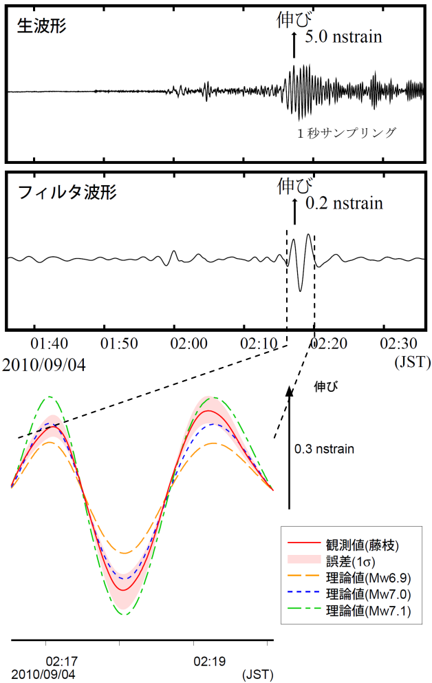
藤枝観測点の観測波形と理論波形の振幅比較（上図）
