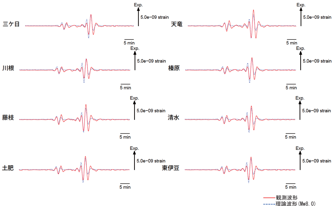
理論波形と体積歪観測点 8 カ所の観測波形との比較 データには周期 120～333 秒のバンドパスフィルタを時間軸の正逆両方向にかけている。
