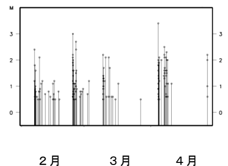
領域a内のM-T図 (2016年2月1日～4月28日、 M≥0.5、深さ0～20km)
