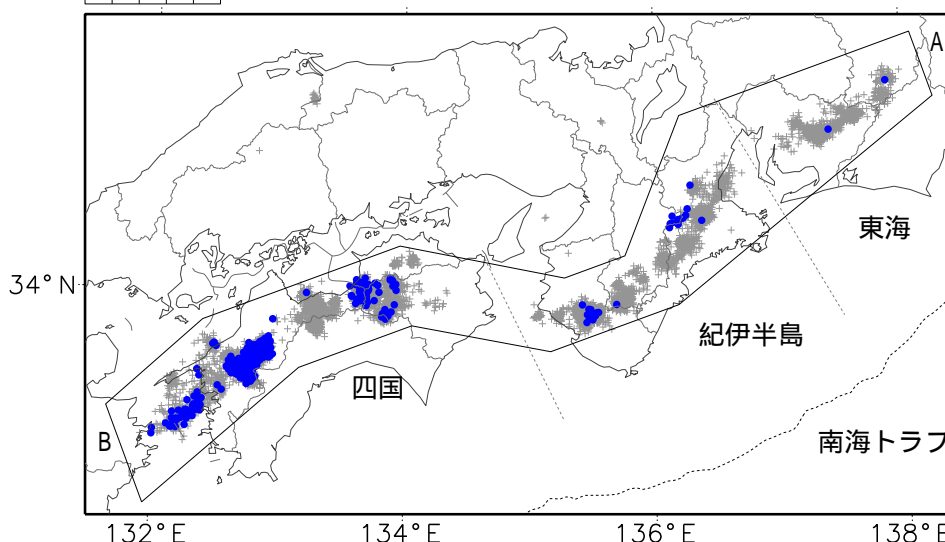
震央分布図（2023年04月26日～2024年04月25日：過去1年間、M全て、深さ全て） 2024年04月19日以降の震源を青く表示
