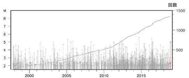
領域b内の地震活動経過図及び回数積算図
