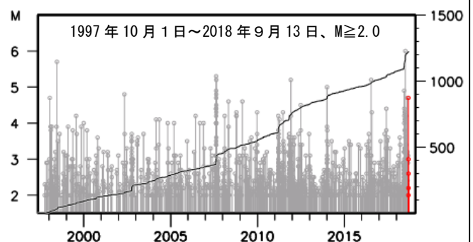
領域a内の地震活動経過図及び回数積算図 * 2018年9月7日以降の地震を赤で表示
