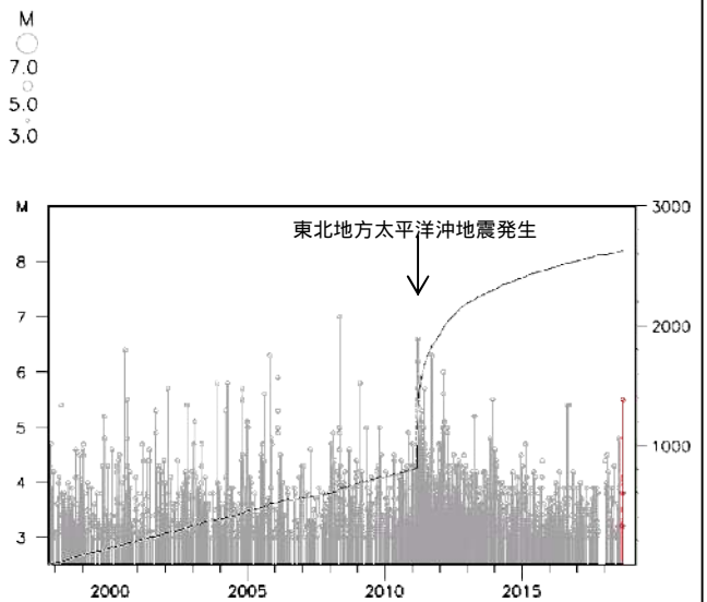
領域a内の地震活動経過図及び回数積算図
