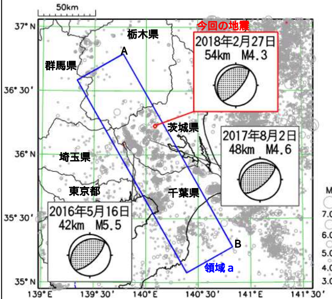
震央分布図
