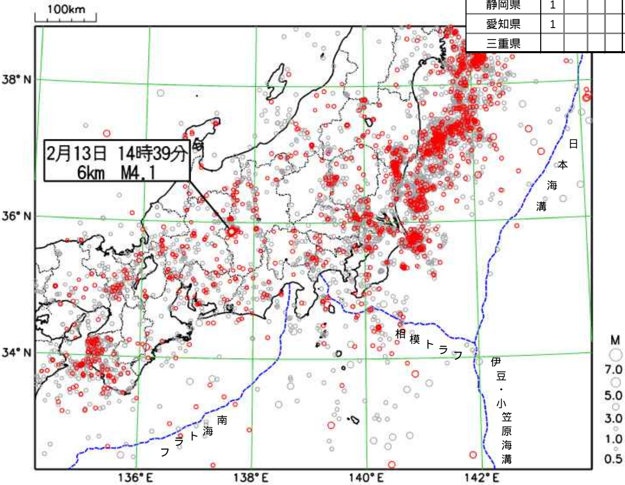
震央分布図
