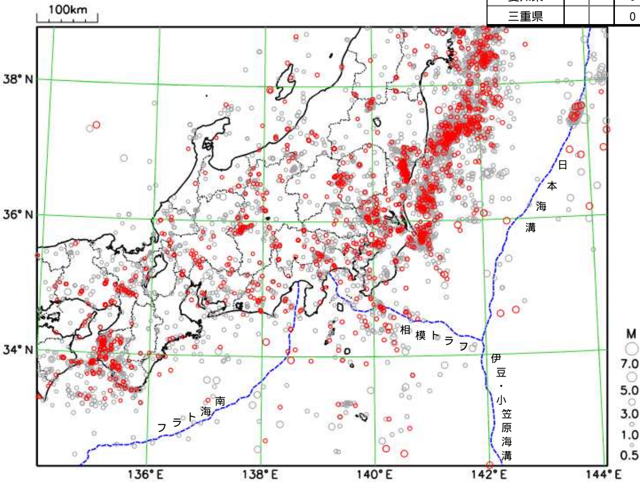
震央分布図
