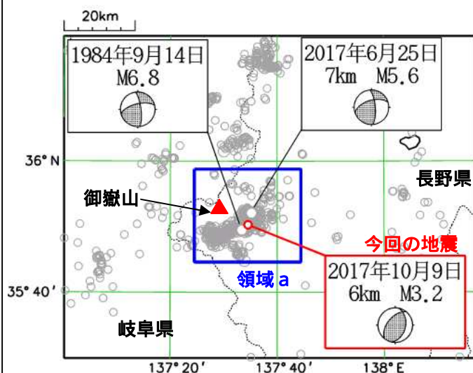
震央分布図
