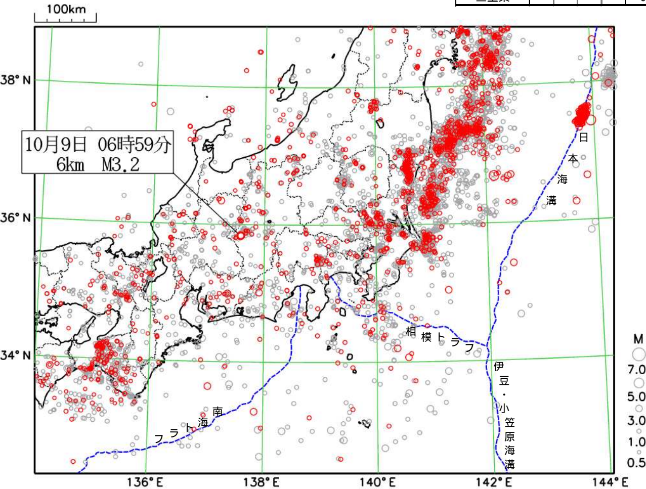
震央分布図
