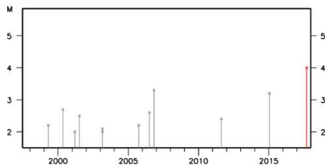
領域b内の地震活動経過図
