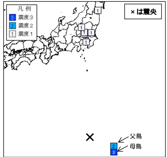
震度分布図 震度分布図は各観測点の震度を表しています。
