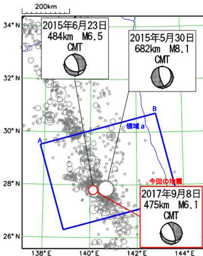
震央分布図 (1997 年 10 月 1 日 ~ 2017 年 9 月 14 日、深さ 100 ~ 700km、M 4.0) 2017 年 9 月 8 日以降の地震を赤で表示
