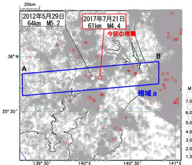
震央分布図
