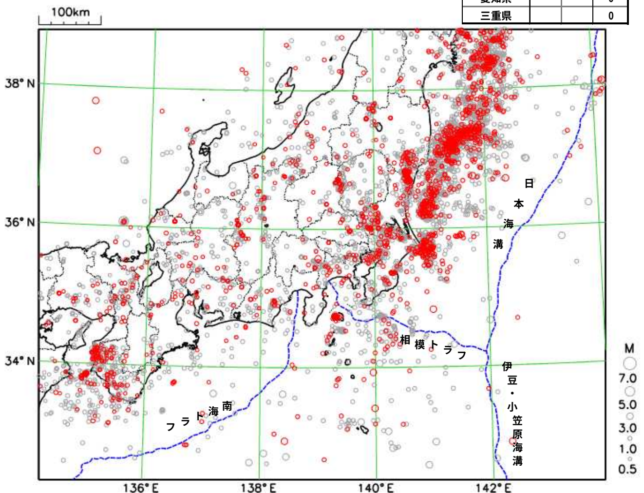
震央分布図
