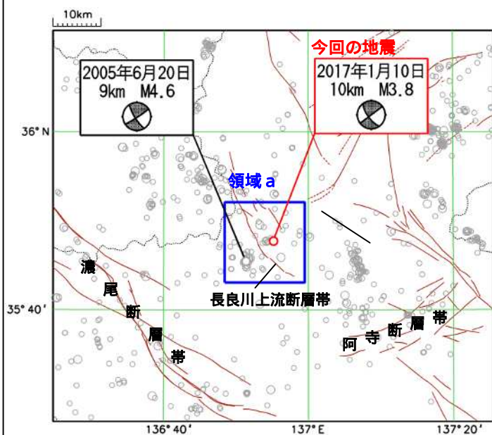
震央分布図
