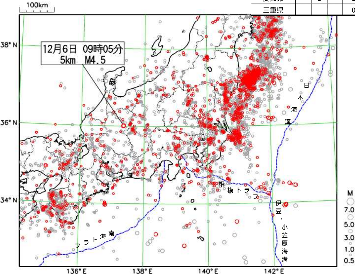
震央分布図
