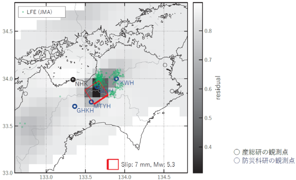
(b1) 推定された断層モデル
