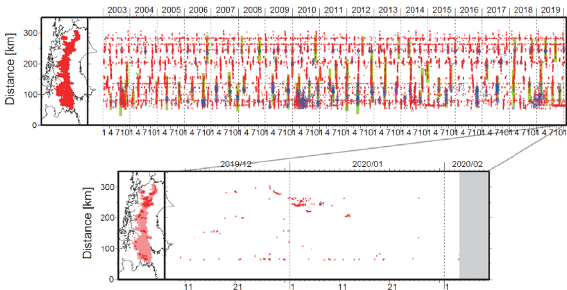
図1. 四国における2003年1月～2020年2月3日までの深部低周波微動の時空間分布(上図)。赤丸はエンベロープ相関・振幅ハイブリッド法 (Maeda and Obara, 2009) およびクラスタ処理 (Obara et al., 2010) によって1時間毎に自動処理された微動分布の重心である。青菱形は周期20秒に卓越する超低周波地震 (Ito et al., 2007) である。黄緑色太線は、これまでに検出された短期的スロースリップイベント (SSE) を示す。下図は2020年1月を中心とした期間の拡大図である。12月27日～1月9日頃には、徳島県東部から愛媛県東部において活発な微動活動がみられた。この活動は徳島県東部において開始したのち、西方向への活動域の移動がみられた。その後、1月1日頃からは徳島・香川・愛媛県境付近において活発化がみられ、4日頃まで西方向への活動域の拡大がみられた。その後活動は低調になりつつ、9日頃まで継続した。これ以外の活動として、1月12日頃には愛媛県東部においてごく小規模な活動がみられた。1月18～19日頃には豊後水道において、小規模な活動がみられた。
