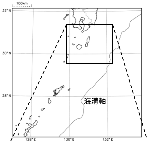
震央分布図 (1997年10月1日～2019年1月31日 深さ0～90km、M≥2.5)
