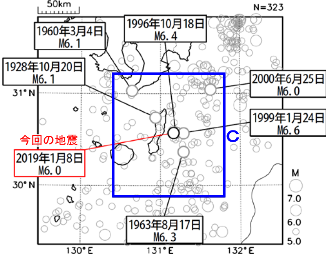
震央分布図 (1923年1月1日～2019年1月31日、 深さ0～200km、M≥5.0)
