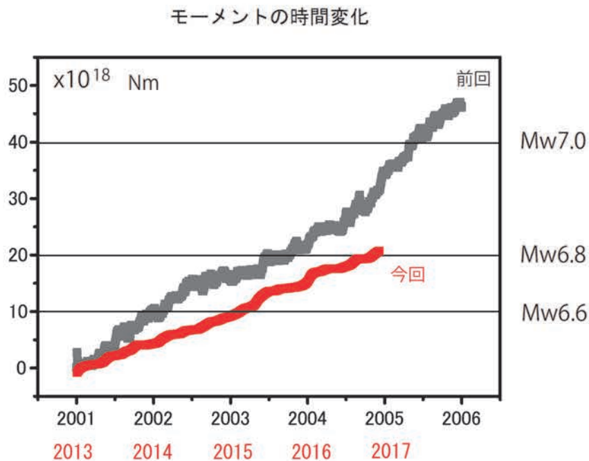
図 16 国土地理院 GNSS 観測結果による、長期的ゆっくりすべりの発生を示唆する非正常地殻変動から推定される累積すべり分布及びモーメントの時間変化の比較
