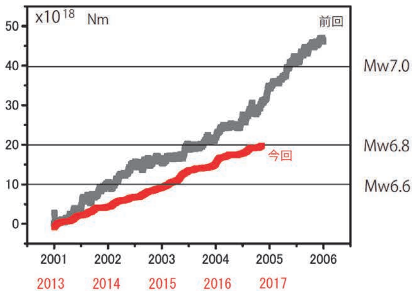
図 17 国土地理院 GNSS 観測結果による、長期的ゆっくりすべりの発生を示唆する非正常地殻変動から推定される累積すべり分布及びモーメントの時間変化の比較
