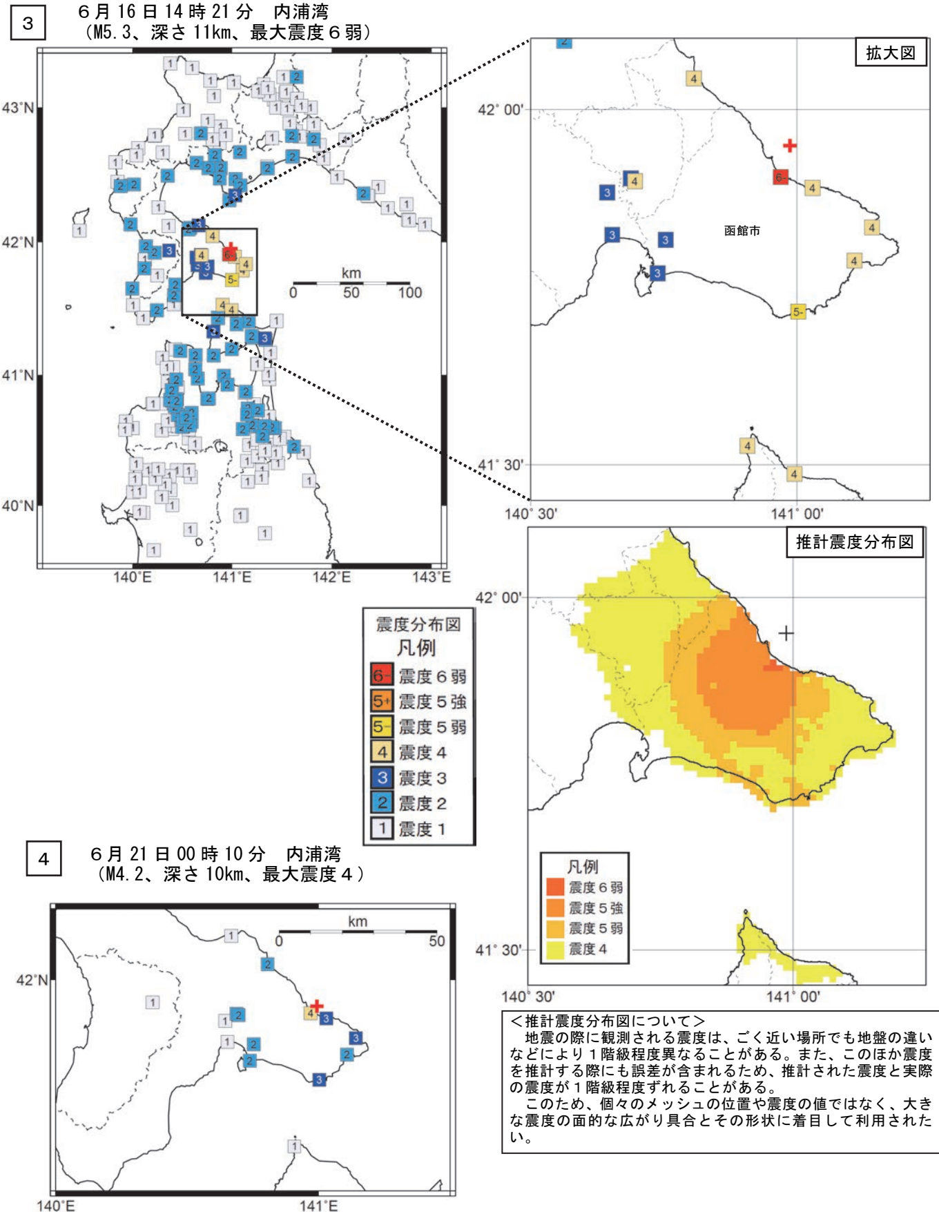
図 3-1 震度分布図（各図の左上の数字は p. 2 の「表 1 平成 28 年 6 月に日本及びその周辺で発生した主な地震」の番号に対応する。+印は震央を示す。）
