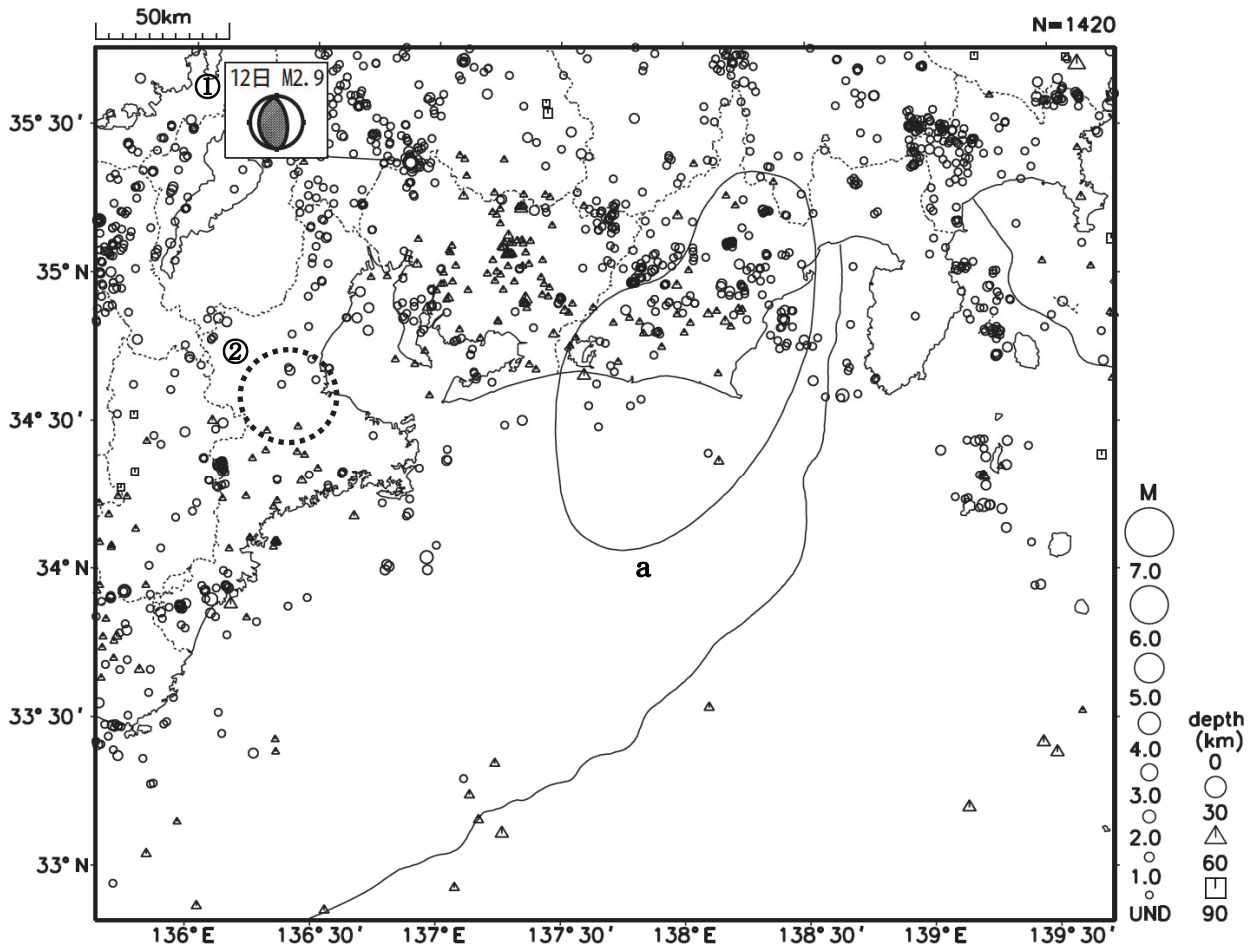
図1 震央分布図（2016年6月1日～30日：深さ0～90km、Mすべて。図中の領域aは東海地震の想定震源域。）
