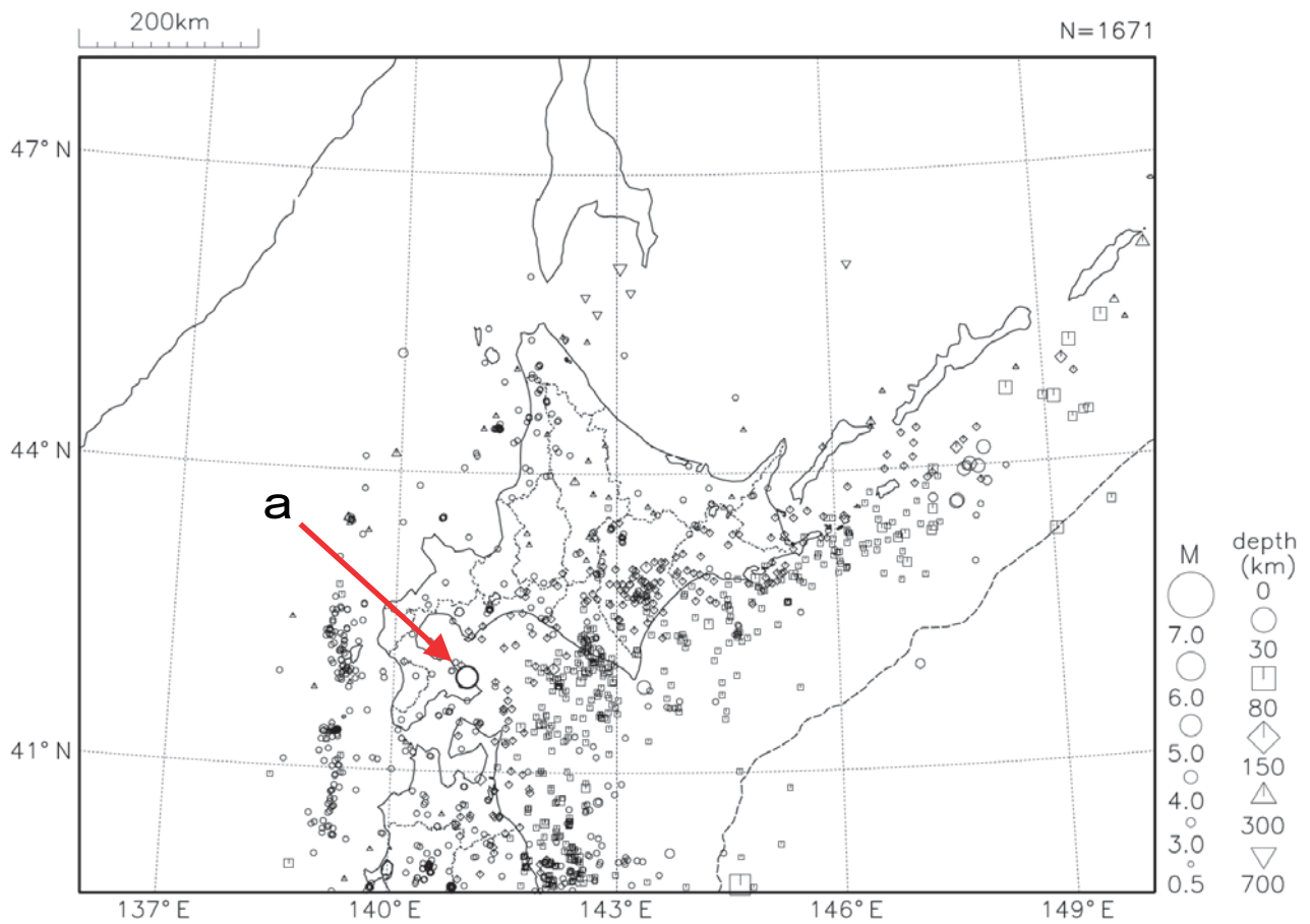
図 4 北海道地方の震央分布図（2016 年 6 月 1 日～6 月 30 日、 M \geq 0.5 ）
