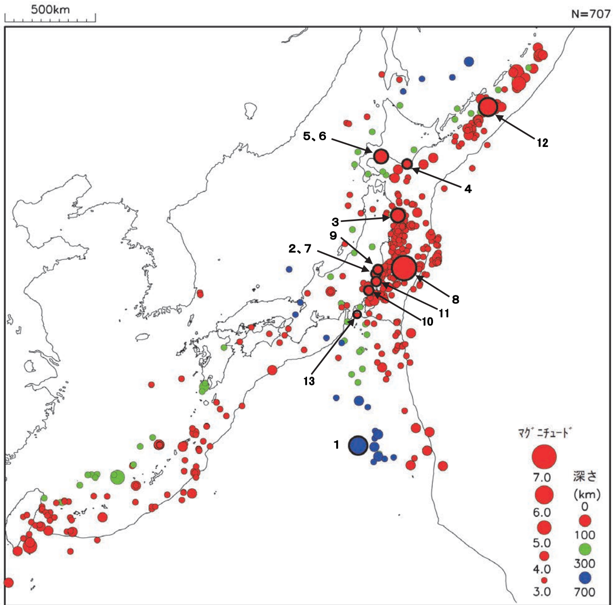
図 2 平成 26 年 7 月に日本及びその周辺で発生した M3.0 以上の地震の震央分布図 (図中の数字は表 1 の番号に対応)
