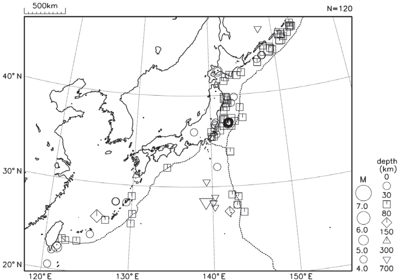
図 1 平成 26 年 7 月に日本及びその周辺で発生した M4.0 以上の地震の震央分布図
