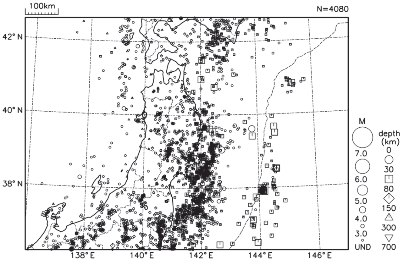
図5 東北地方の震央分布図（2014年5月1日～5月31日）
