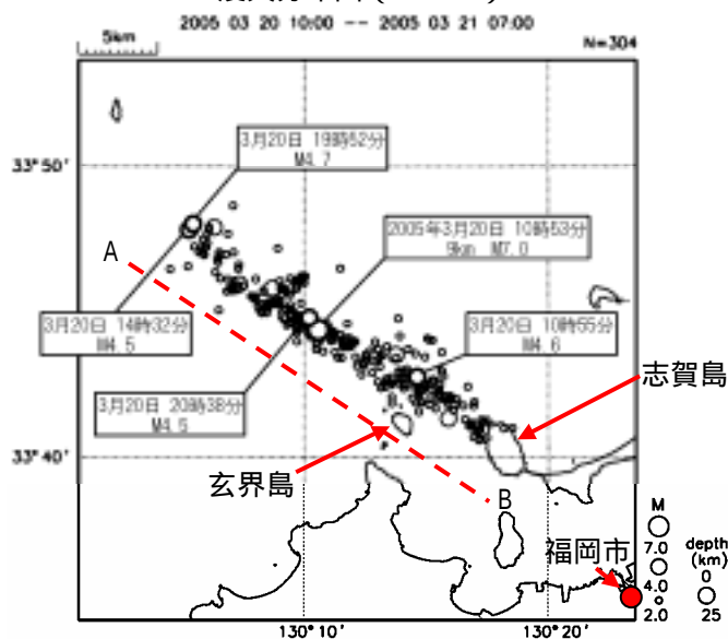
震央分布図 (M 2.0)
