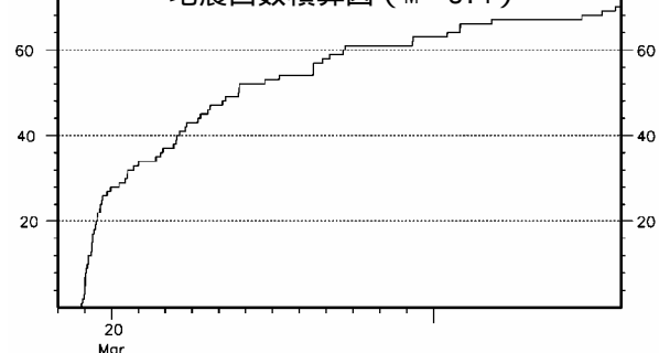
地震回数積算図 (M 3.4)
