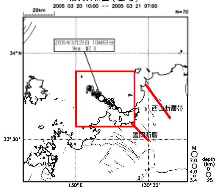
震央分布図 (広域)
