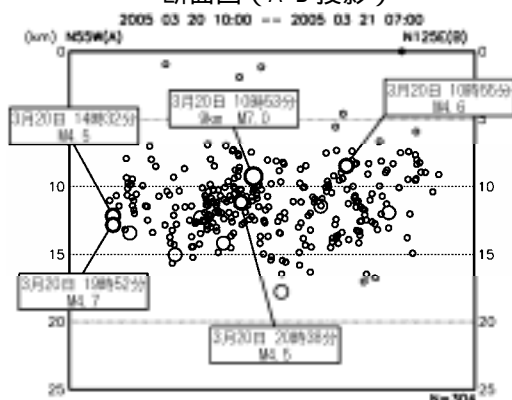
断面図 (A-B 投影)
