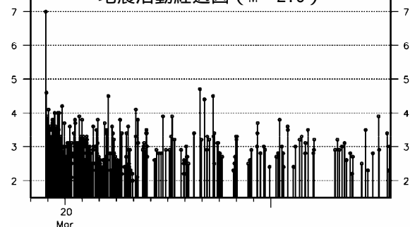
地震活動経過図 (M 2.0)
