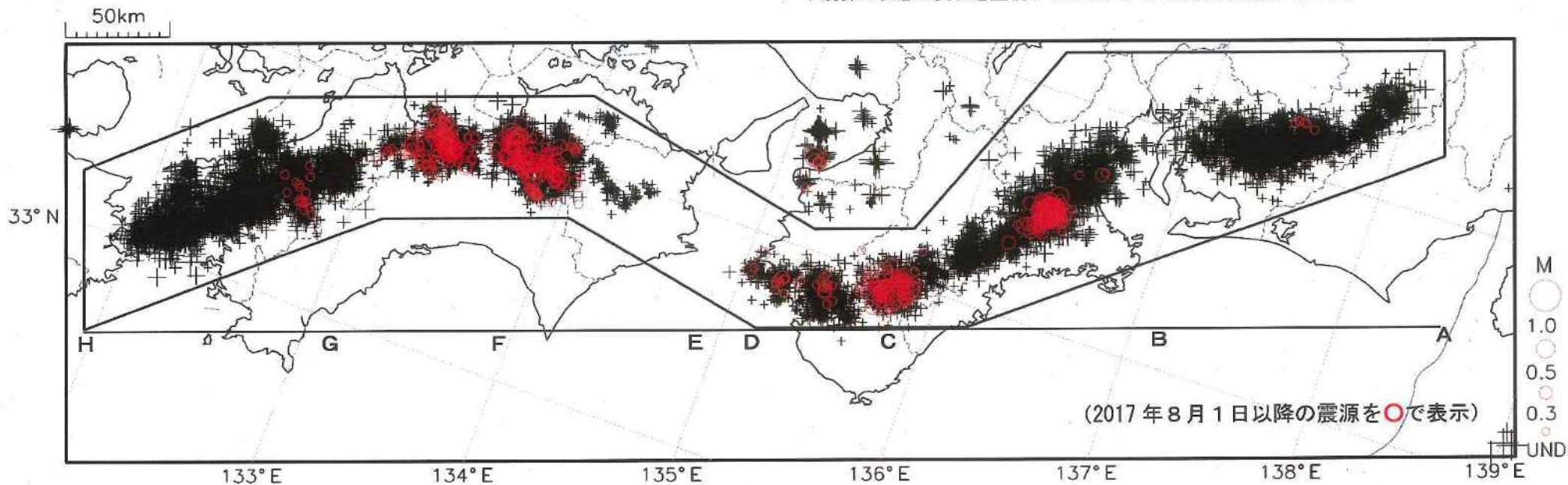
(2017年8月1日~2017年9月19日)
