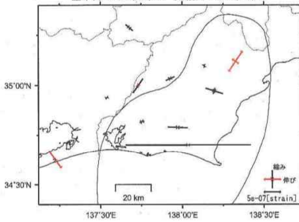
基準日：2016/12/01 比較日：2017/03/01
