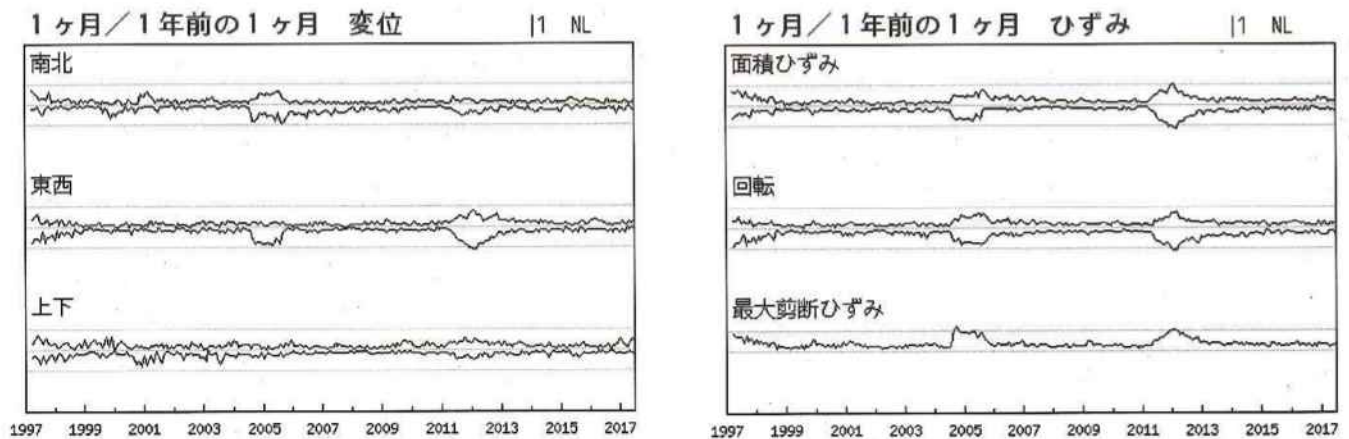
対象範囲内の最大値の経過 (1997年1月～2017年9月)
