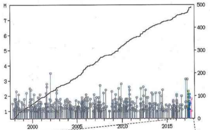
領域b内のMT図・回数積算図
