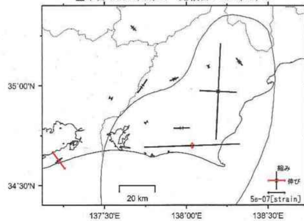
基準日：2017/06/21 比較日：2017/09/19
