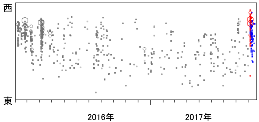
領域b内の時空間分布図 (東西投影)
