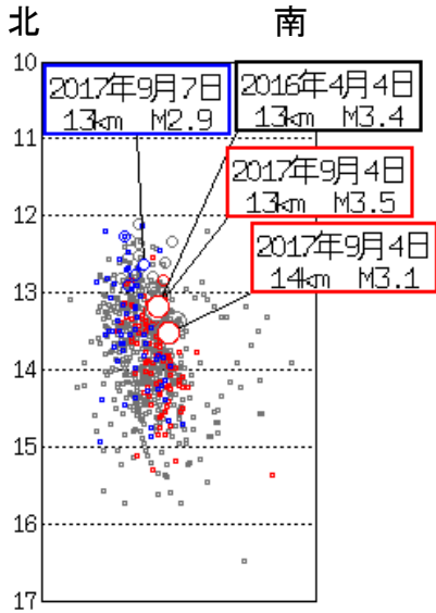
領域b内の断面図 (南北投影)
