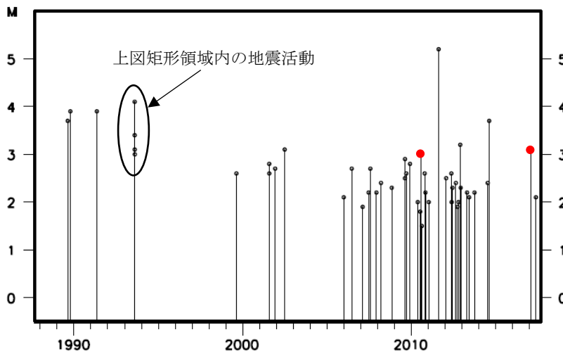
想定震源域内で発生した地震のうち、2010年1月以降に発生したM3.0以上かつプレート境界からの鉛直方向の距離が±3km以内の地震の枠を赤く表示
