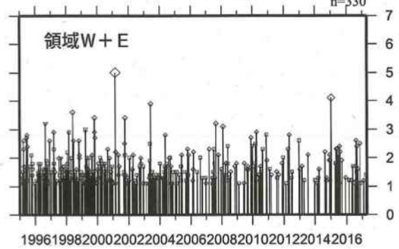
M-T図
