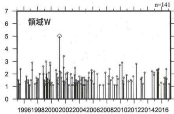
M-T図
