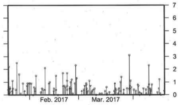
M-T図
