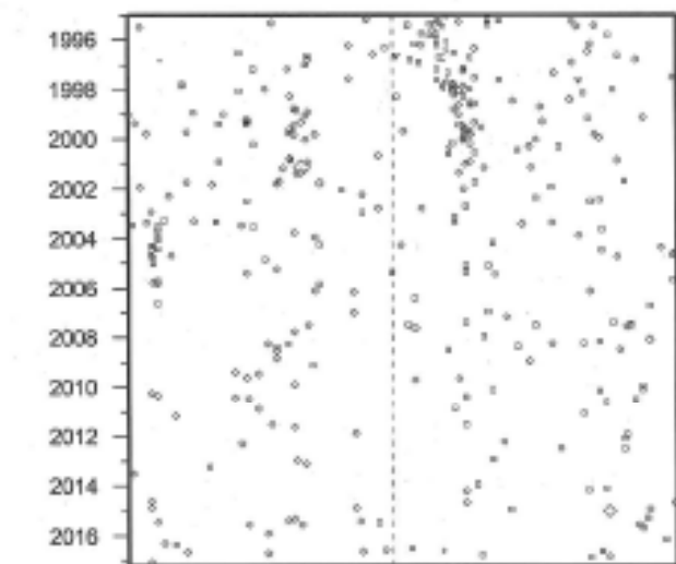
時空間分布図 (東西方向)
