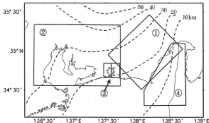
* Hirose et al. (2008) によるプレート境界の等深線を破線です
