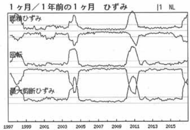
対象範囲内の最大値の経過 (1997年1月~2017年2月)
