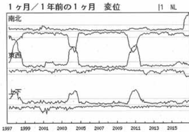
対象範囲内の最大値の経過 (1997年1月~2017年2月)
