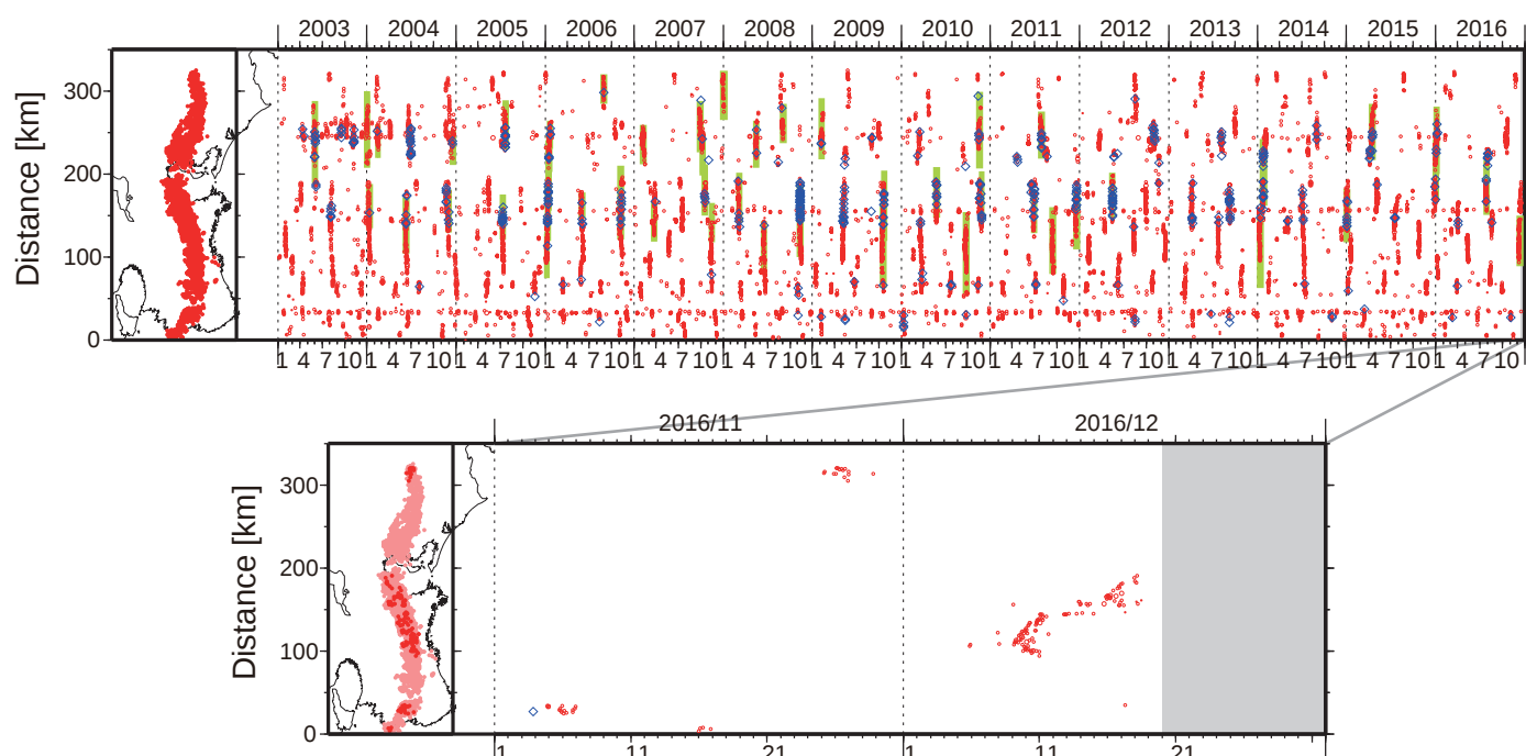
図 1. 紀伊半島・東海地域における 2003 年 1 月 ~ 2016 年 12 月 19 日までの深部低周波微動の時空間分布 (上図). 赤丸はエンベロップ相関・振幅ハイブリッド法 (Maeda and Obara, 2009) およびクラスタ処理 (Obara et al., 2010) によって 1 時間毎に自動処理された微動分布の重心である. 青菱形は周期 20 秒に卓越する超低周波地震 (Ito et al., 2007) である. 黄緑色の太線はこれまでに検出された短期的スロースリップイベント (SSE) を示す. 下図は 2016 年 11 ~ 12 月の拡大図である. 11 月下旬以降については、12 月 5 ~ 18 日頃に、奈良県中部の三重県境付近から三重県中部にかけての領域で、活発な活動がみられた. この活動は三重・奈良県境付近で開始し、当初は低調であったが、9 日 2:38 頃 (JST) に、ソロモン諸島で Mw7.8(USGS) の地震が発生した後、3 時台から沈み込むプレートの浅い側で活動が活発化し、北東・南西方向への活動域の移動がみられた. 北東側の活動は弱まりながらも継続した後、16 日頃から活発化し、18 日頃まで主に北東方向に広がりつつ継続した. この領域での顕著な活動は 2016 年 8 月以来であり、活動に伴い短期的 SSE の断層モデルも推定されている. 11 月 25 ~ 27 日頃には長野県南部で小規模な活動がみられた.
