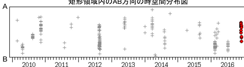
矩形領域内のAB方向の時空間分布図
