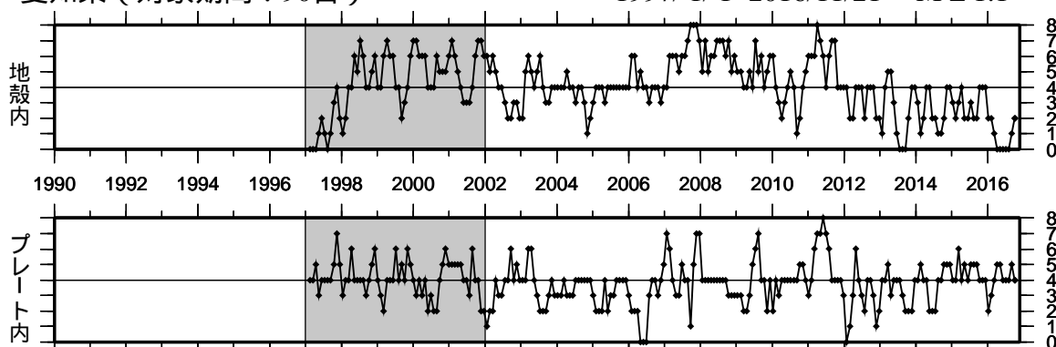
② 愛知県（対象期間：90日） 1997/ 1/ 1~2016/11/21 M ≥ 1.1
