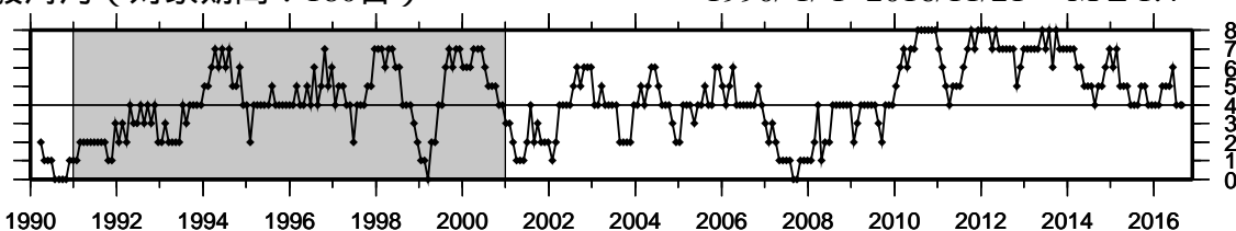
④ 駿河湾（対象期間：180日） 1990/ 1/ 1~2016/11/21 M ≥ 1.4
