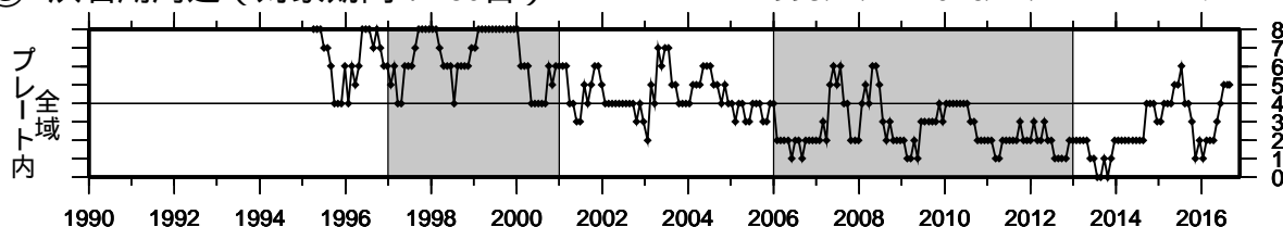
④ 駿河湾（対象期間：180日） 1990/ 1/ 1~2016/11/21 M ≥ 1.4
