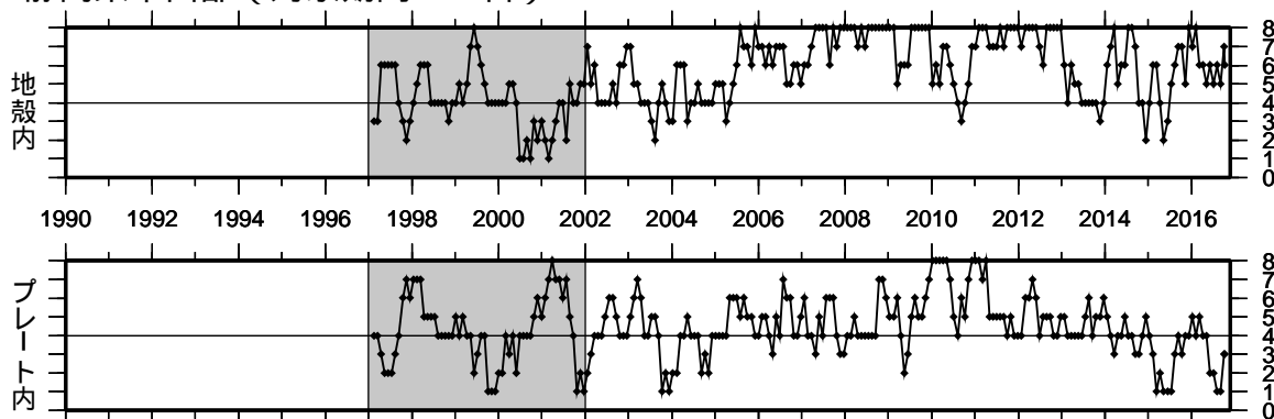
① 静岡県中西部（対象期間：90日） 1997/ 1/ 1~2016/11/21 M ≥ 1.1
