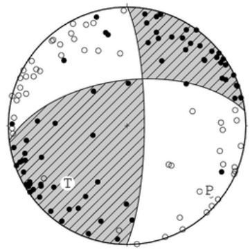
今回の地震の発震機構解(自動解)
