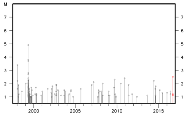
領域b内MT図
