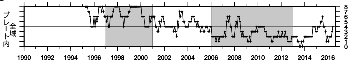
④ 駿河湾（対象期間：180日） 1990/1/1~2016/8/23 M ≥ 1.4
