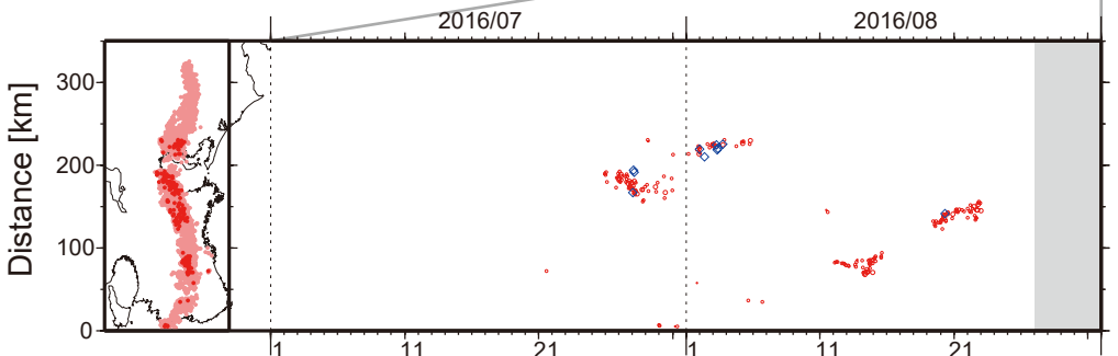
図1. 紀伊半島・東海地域における2003年1月～2016年8月26日までの深部低周波微動の時空間分布(上図). 赤丸はエンベロープ相関・振幅ハイブリッド法 (Maeda and Obara, 2009) およびクラスタ処理 (Obara et al., 2010) によって1時間毎に自動処理された微動分布の重心である. 青菱形は周期20秒に卓越する超低周波地震 (Ito et al., 2007) である. 黄緑色の太線はこれまでに検出された短期的スロースリップイベント (SSE) を示す. 下図は2016年7～8月の拡大図である.
