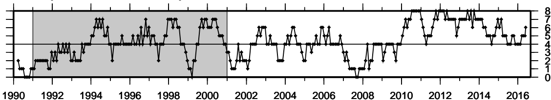
④ 駿河湾（対象期間：180日） 1990/1/1~2016/8/23 M ≥ 1.4
