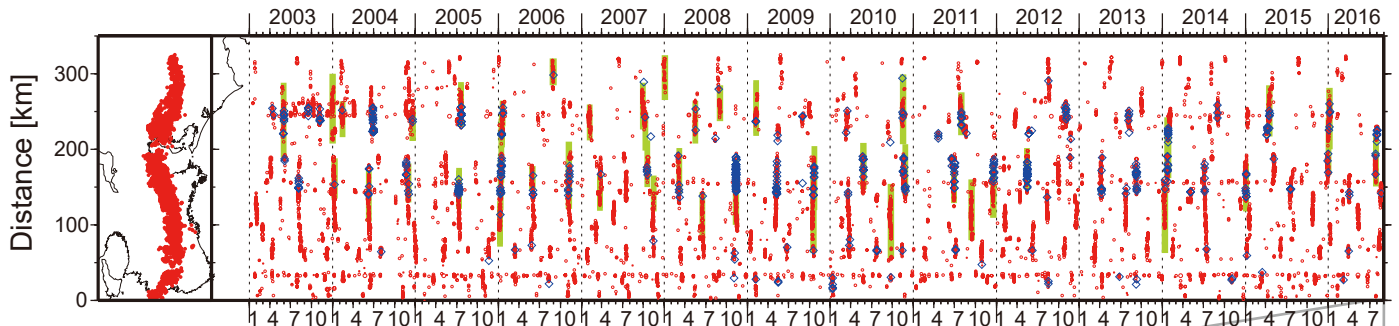
図1. 紀伊半島・東海地域における2003年1月～2016年8月26日までの深部低周波微動の時空間分布(上図). 赤丸はエンベロープ相関・振幅ハイブリッド法 (Maeda and Obara, 2009) およびクラスタ処理 (Obara et al., 2010) によって1時間毎に自動処理された微動分布の重心である. 青菱形は周期20秒に卓越する超低周波地震 (Ito et al., 2007) である. 黄緑色の太線はこれまでに検出された短期的スロースリップイベント (SSE) を示す. 下図は2016年7～8月の拡大図である.
