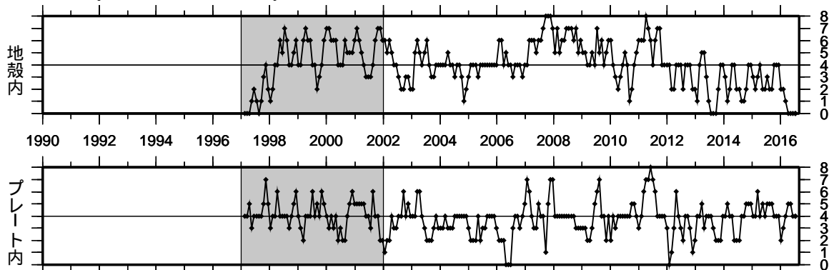
② 愛知県（対象期間：90日） 1997/1/1~2016/8/23 M ≥ 1.1
