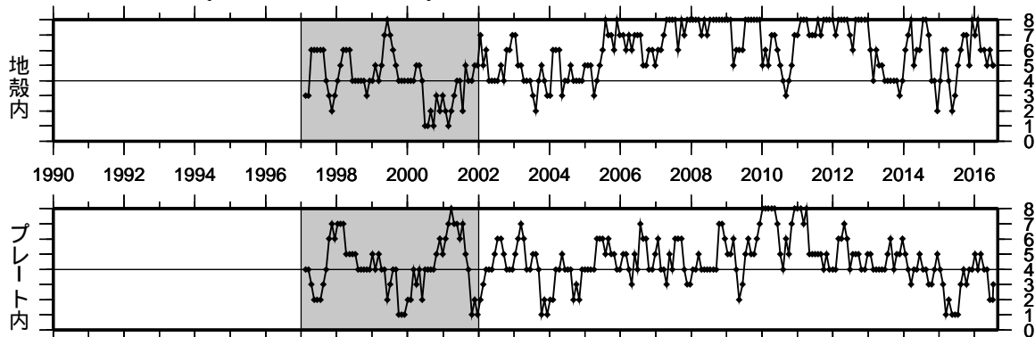
① 静岡県中西部（対象期間：90日） 1997/1/1~2016/8/23 M ≥ 1.1
