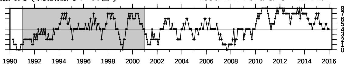
④ 駿河湾（対象期間：180日） 1990/ 1/ 1~2016/ 3/23 M ≥ 1.4
