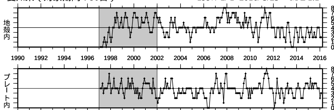
② 愛知県（対象期間：90日） 1997/ 1/ 1~2016/ 3/23 M ≥ 1.1
