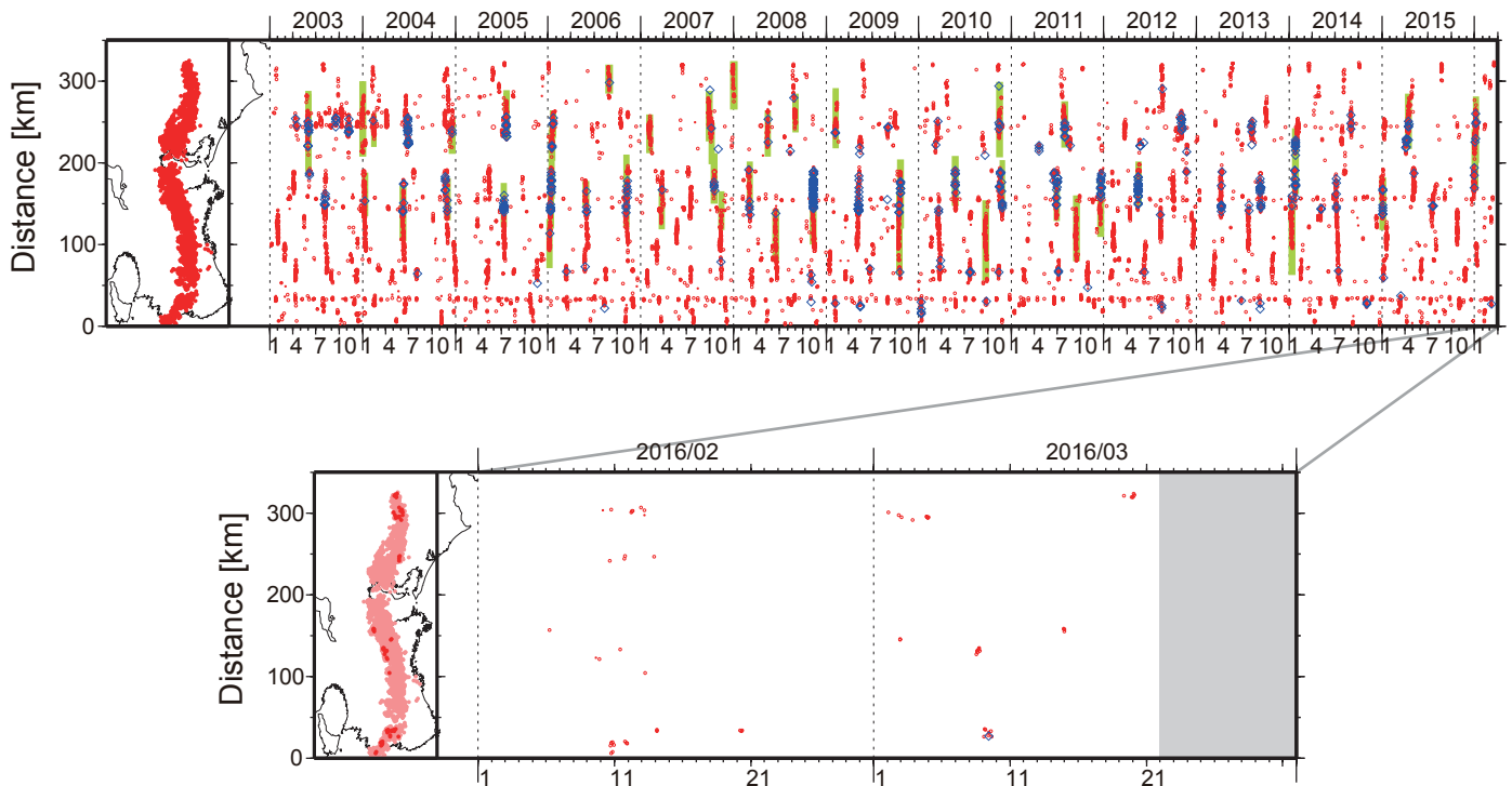
図 1. 紀伊半島・東海地域における 2003 年 1 月～2016 年 3 月 21 日までの深部低周波微動の時空間分布 (上図)．赤丸はエンベロープ相関・振幅ハイブリッド法 (Maeda and Obara, 2009) およびクラスター処理 (Obara et al., 2010) によって 1 時間毎に自動処理された微動分布の重心である．青菱形は周期 20 秒に卓越する超低周波地震 (Ito et al., 2007) である．黄緑色の太線はこれまでに検出された短期的スロースリップイベント (SSE) を示す．下図は 2016 年 2～3 月の拡大図である 2 月後半以降、顕著な活動は特にみられなかったものの、2 月 20 日頃には和歌山県中部で、3 月 2～5 日頃には長野県南部で、3 月 8 日頃には三重・奈良県境付近で、3 月 9 日頃には和歌山県中部で、3 月 14～15 日頃には三重県北部で、それぞれごく小規模な活動がみられた．3 月 19～20 日頃には長野県南部の 3 月 2～5 日の活動域の北側で、ごく小規模な活動がみられた．3 月 2 日 21:49 頃 (JST) にスマトラ南西沖で発生した Mw7.8 の地震後には、三重県中部で微動活動が一時的にみられた．
