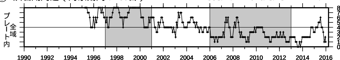
④ 駿河湾（対象期間：180日） 1990/ 1/ 1~2016/ 3/23 M ≥ 1.4
