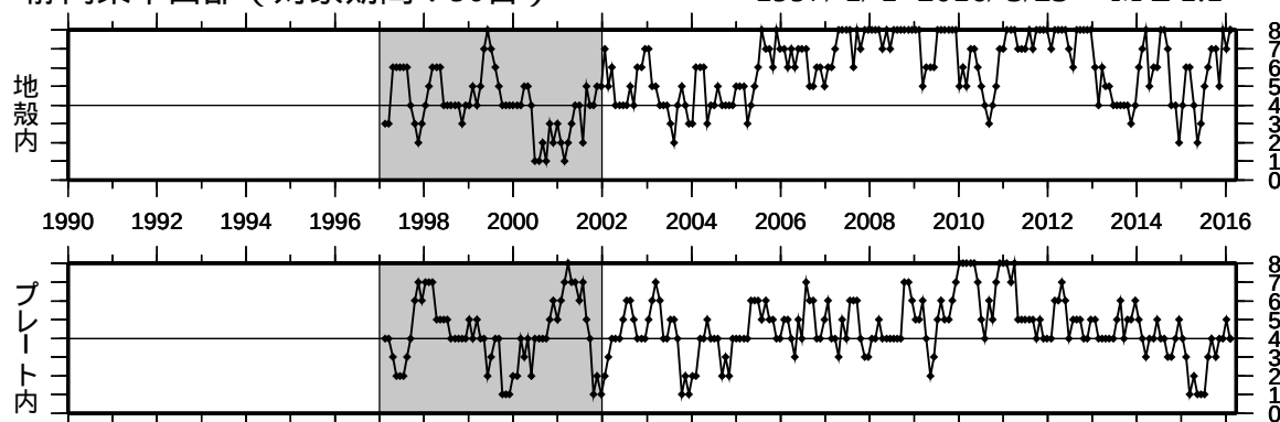
① 静岡県中西部（対象期間：90日） 1997/ 1/ 1~2016/ 3/23 M ≥ 1.1
