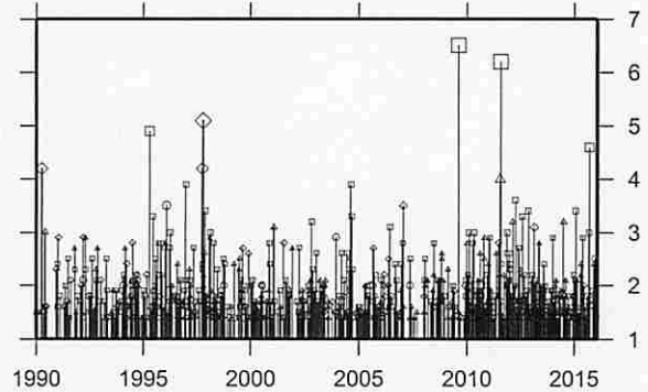
M-I-T図
