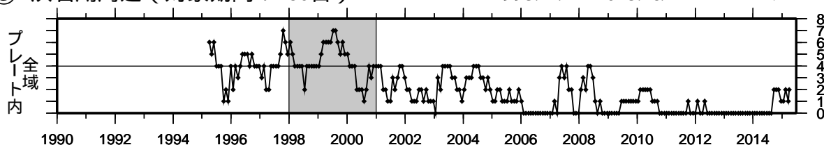
④ 駿河湾（対象期間：180日） 1990/1/1~2015/6/24 M ≥ 1.4
