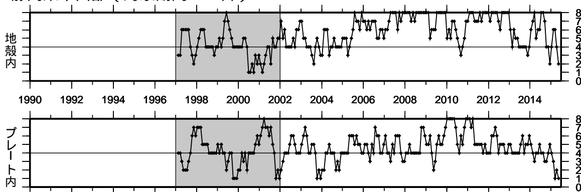
① 静岡県中西部（対象期間：90日） 1997/1/1~2015/6/24 M ≥ 1.1
