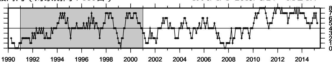
④ 駿河湾（対象期間：180日） 1990/1/1~2015/6/24 M ≥ 1.4
