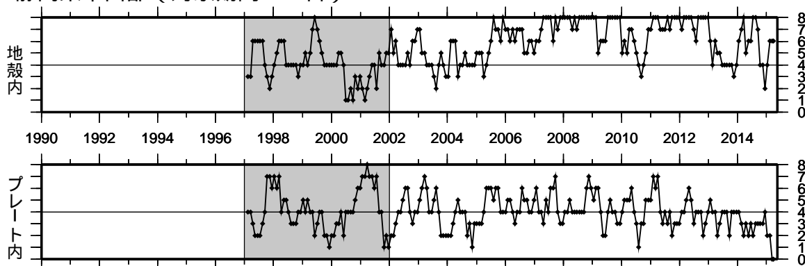
① 静岡県中西部（対象期間：90日） 1997/1/1~2015/5/13 M ≥ 1.1
