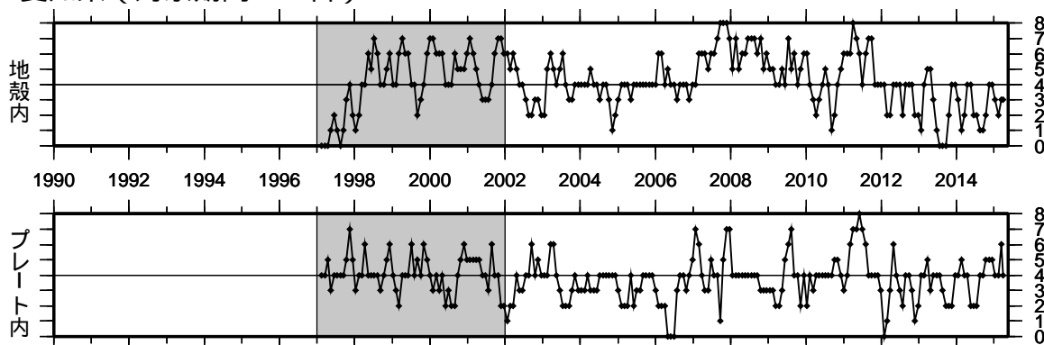
② 愛知県（対象期間：90日） 1997/1/1~2015/5/13 M ≥ 1.1
