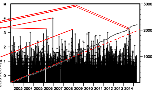
回数積算図とM-T図
