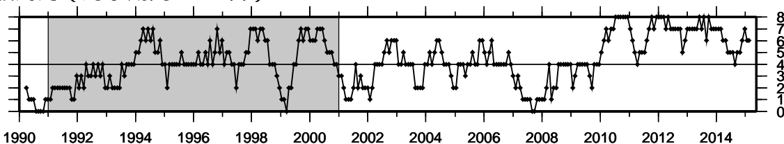
④ 駿河湾（対象期間：180日） 1990/1/1~2015/5/13 M ≥ 1.4
