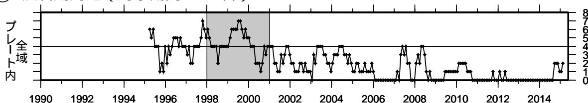
④ 駿河湾（対象期間：180日） 1990/1/1~2015/5/13 M ≥ 1.4
