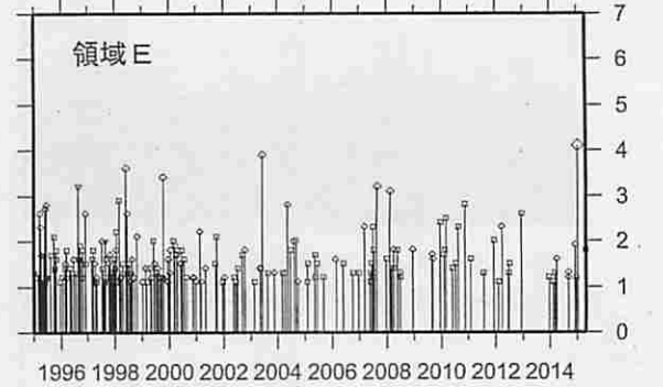
M-T図
