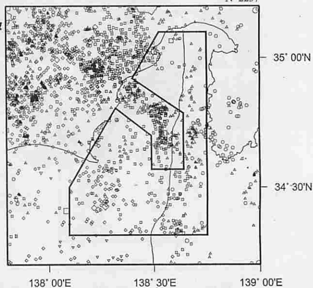
震央分布図
