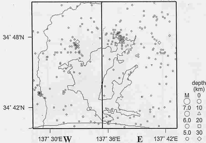
震央分布図
