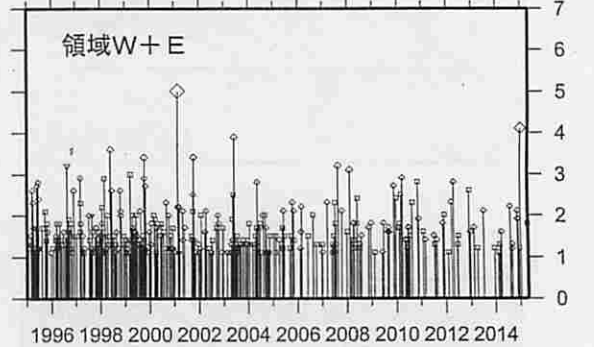
M-T図
