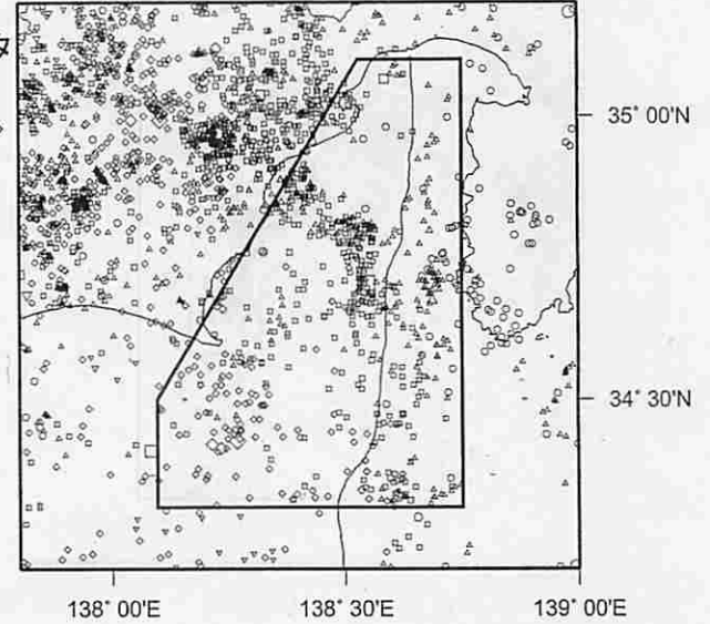
震央分布図
