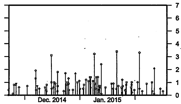
M-T図
