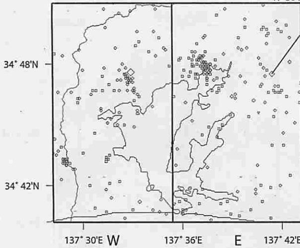
震央分布図
