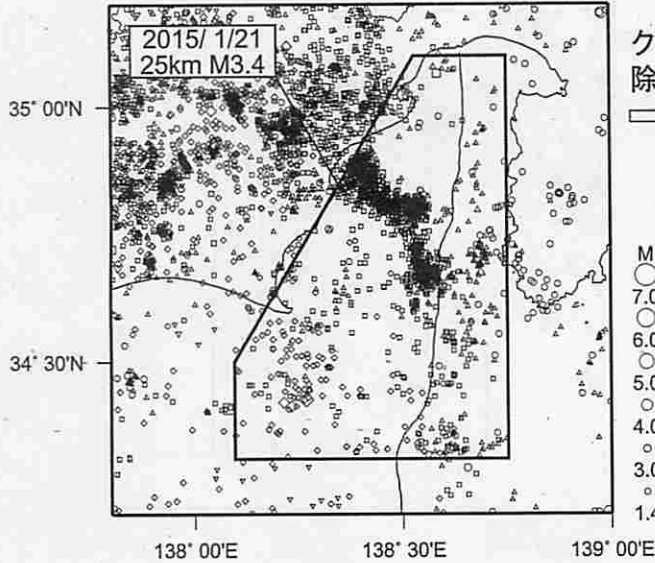
震央分布図
