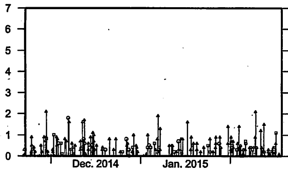
M-T図
