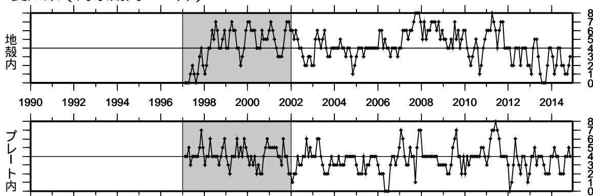
② 愛知県 (対象期間: 90日) 1997/1/1~2014/12/17 M ≥ 1.1
