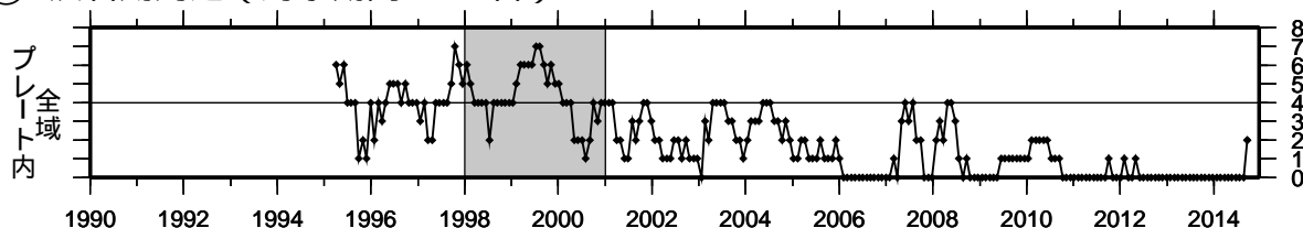
④ 駿河湾 (対象期間: 180日) 1990/1/1~2014/12/17 M ≥ 1.4
