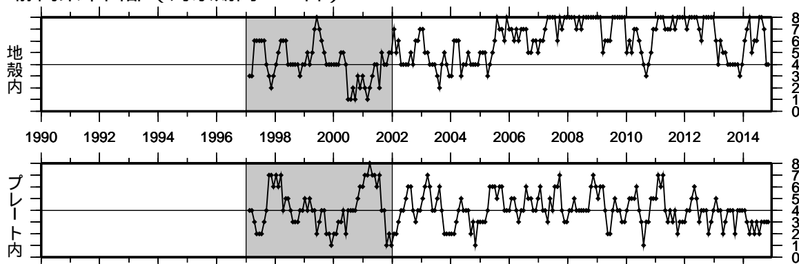
① 静岡県中西部 (対象期間: 90日) 1997/1/1~2014/12/17 M ≥ 1.1
