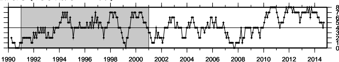
④ 駿河湾 (対象期間: 180日) 1990/1/1~2014/12/17 M ≥ 1.4
