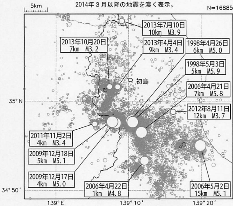
震央分布図（1997年10月1日～2014年4月16日、 M \geq 0.5 、深さ0～20km）
