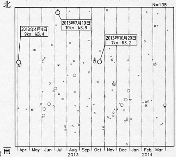
左図内の地震の時空間分布図（南北投影） （2013年4月1日～2014年4月16日）
