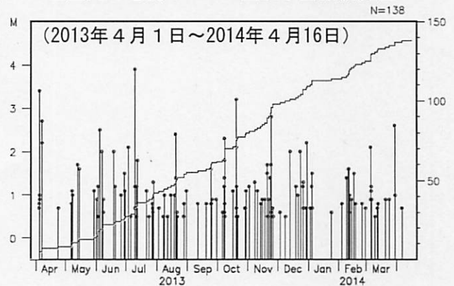
左図内の地震のM-T図及び回数積算図
