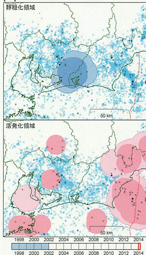
[ 3 ] 2013/12/19--2014/03/18
