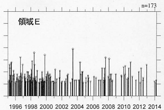
領域E
