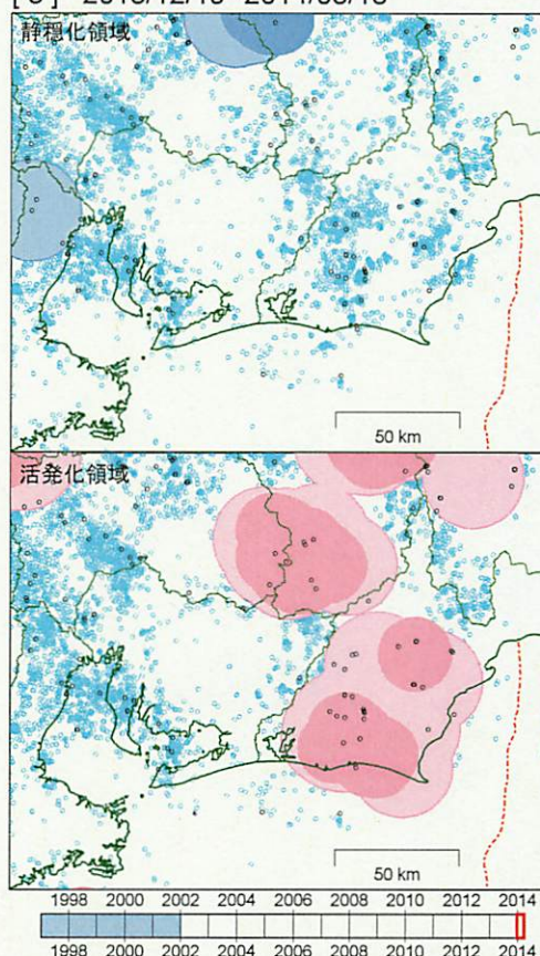
[ 3 ] 2013/12/19--2014/03/18
