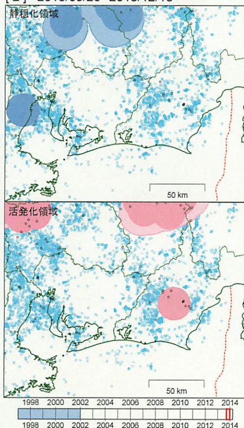
[ 2 ] 2013/09/20--2013/12/18
