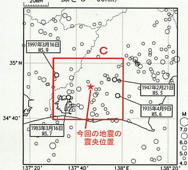
震央分布図
