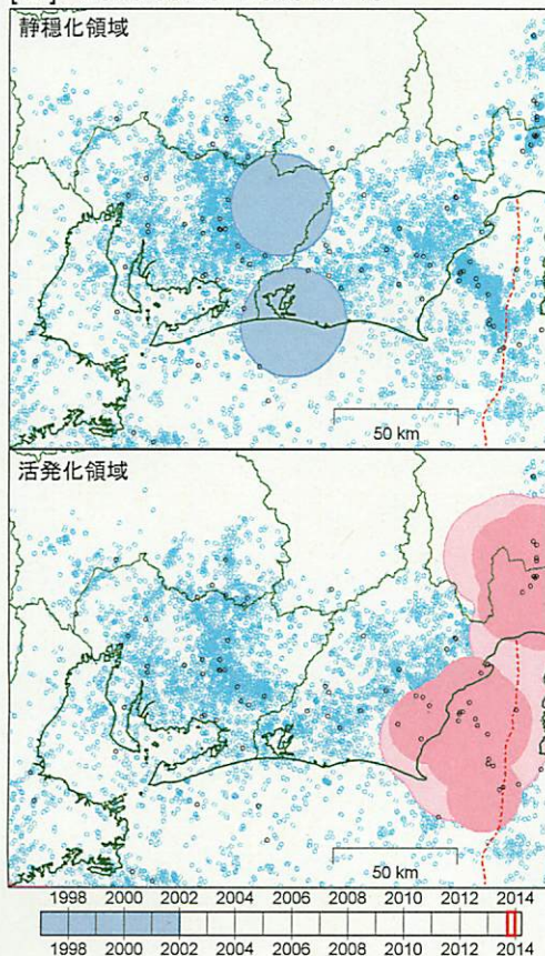
[ 2 ] 2013/09/20--2013/12/18
