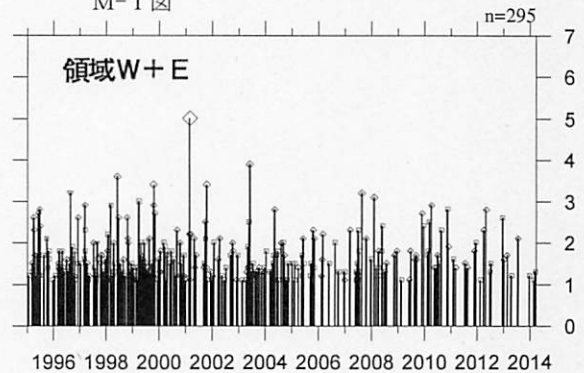
M-T図
