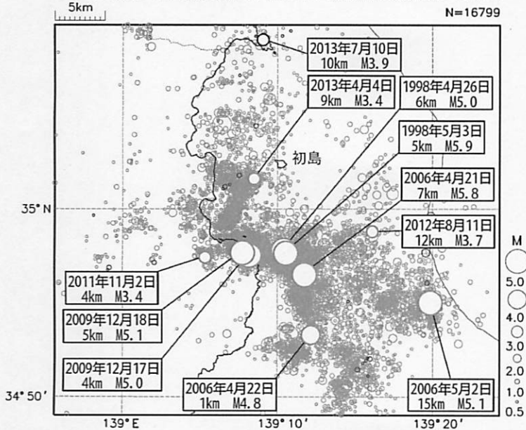
震央分布図（1997年10月1日～2013年8月26日、 M \geq 0.5 、深さ0～20km）
