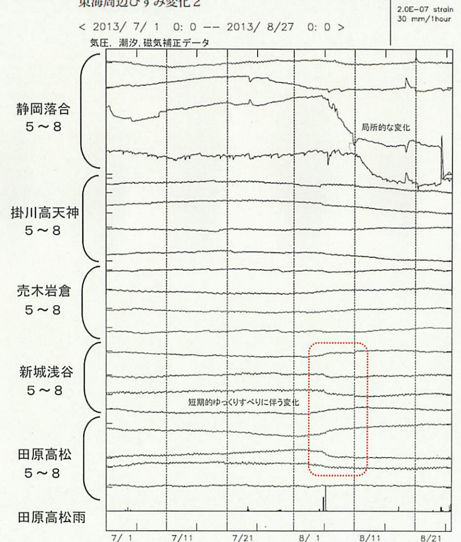
東海周辺ひずみ変化 2
