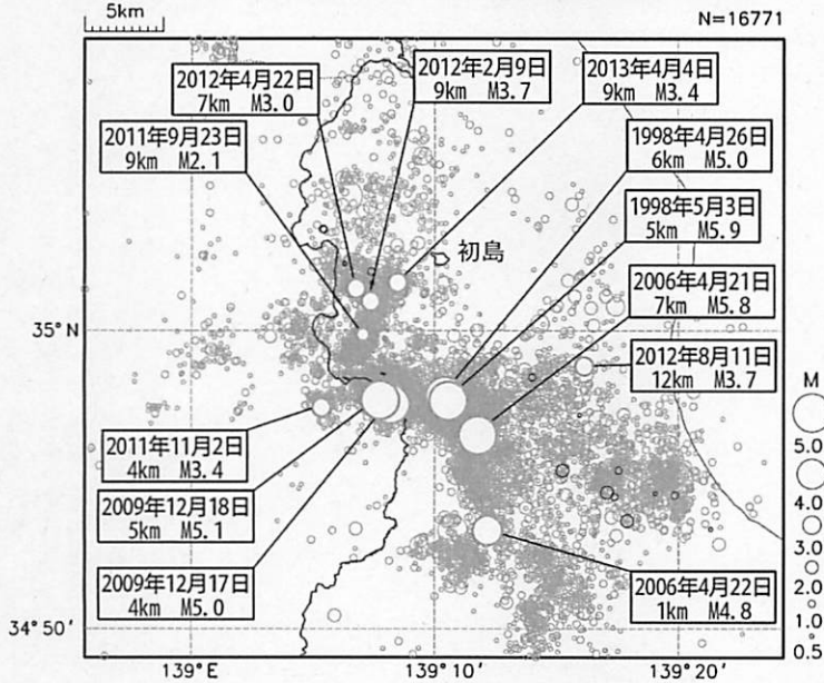
震央分布図（1997年10月1日～2013年6月19日、 M \geq 0.5 、深さ0～20km）
