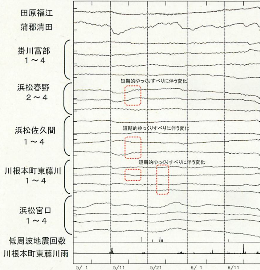
東海周辺ひずみ変化 1
