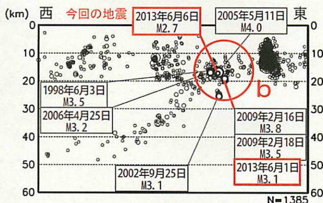
領域a内の断面図（東西投影）
