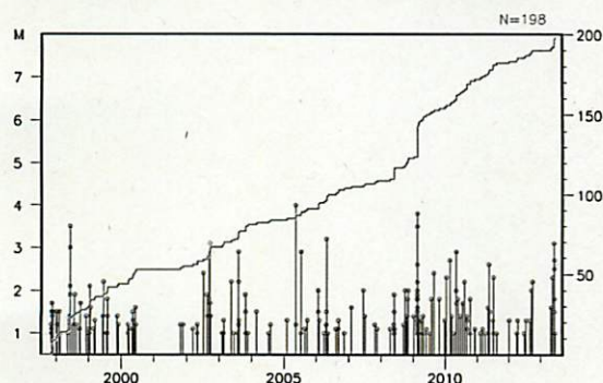
領域b内のM-T図及び地震回数積算図
