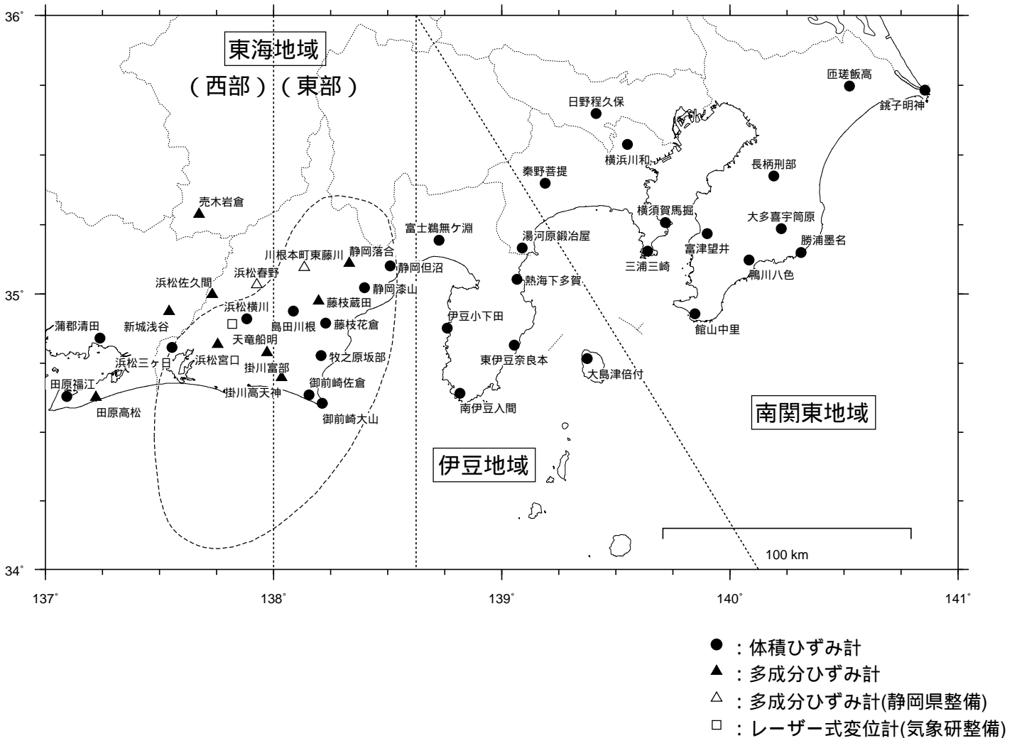
ひずみ計の配置図
