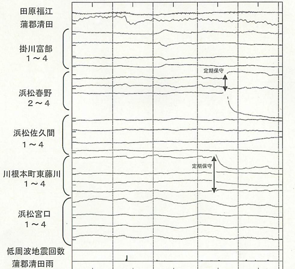
東海周辺ひずみ変化 1
