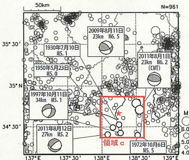
震央分布図 (1923年1月1日~2013年2月20日、 M \geq 4.0 、深さ0~60km)
