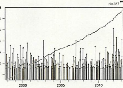
領域b内のM-T図、回数積算図
