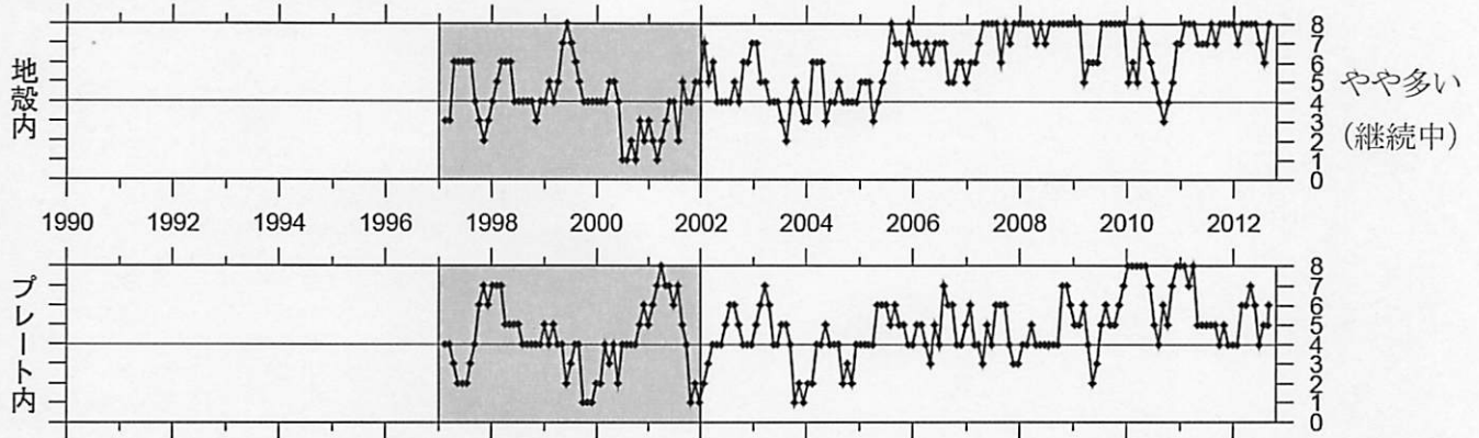
① 静岡県中西部（対象期間：90日）
