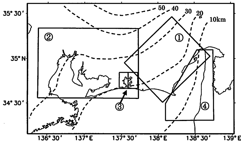
* Hirose et al. (2008) によるプレート境界の等深線を波線で示す
