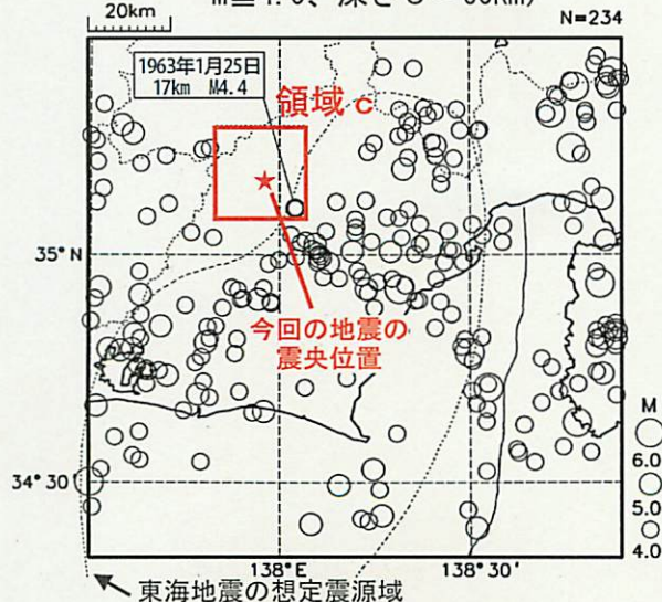
震央分布図 (1923年1月1日~2012年10月17日、 M \geq 4.0 、深さ0~60km)
