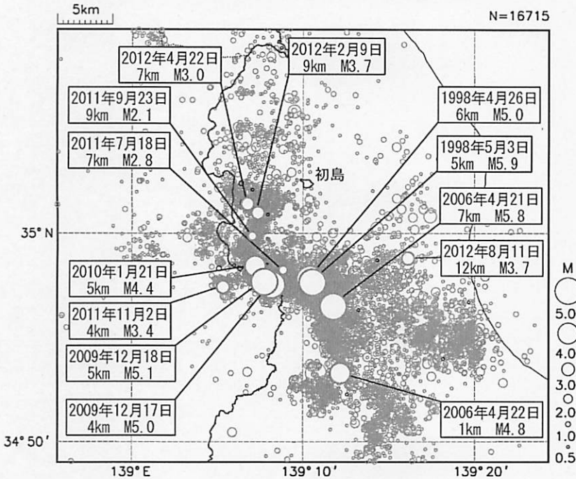
震央分布図（1997年10月1日～2012年10月17日、 M \geq 0.5 、深さ0～20km）
