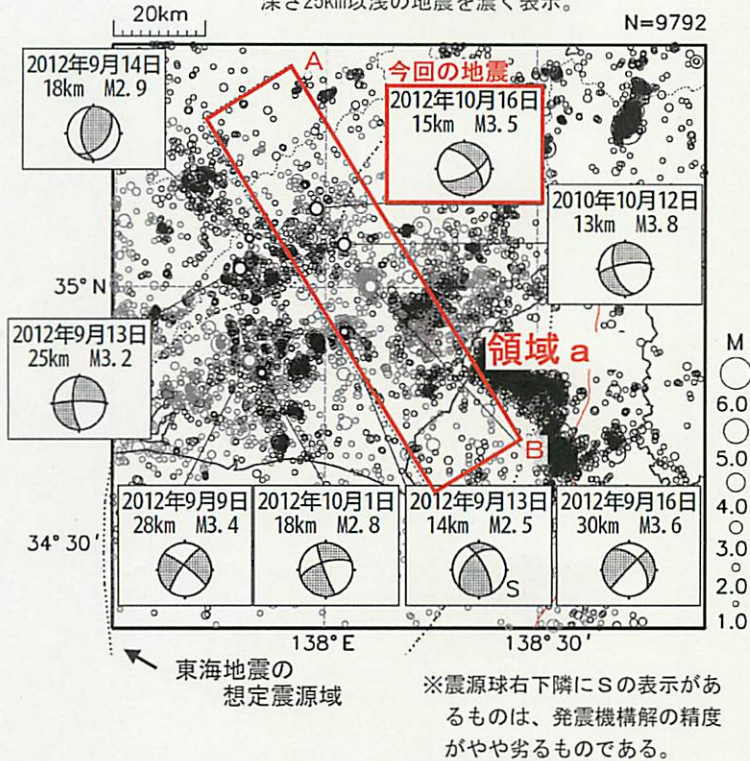
震央分布図 (197年10月1日~2012年10月17日、 M \geq 1.0 、深さ0~60km) 深さ25km以浅の地震を濃く表示。
