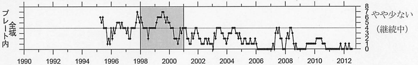
④ 駿河湾（対象期間：180日）
